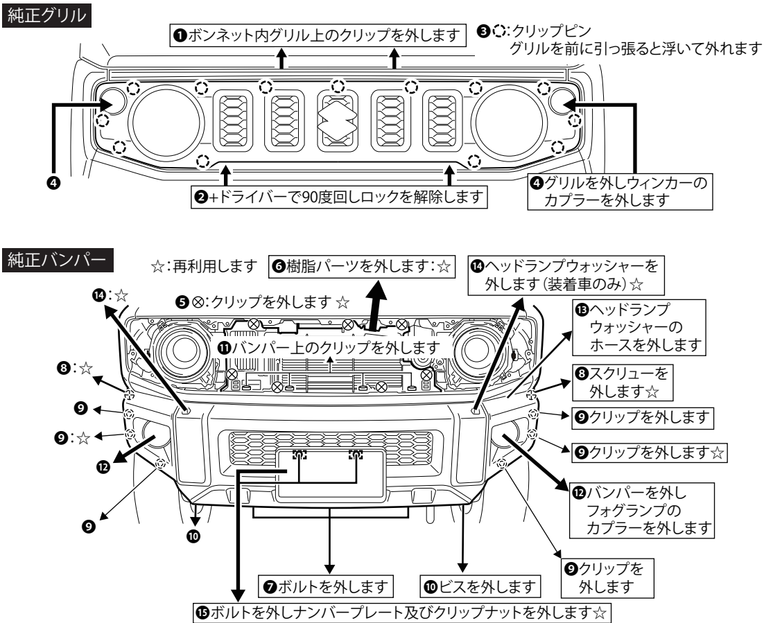
図1 純正グリル及びバンパーの取外し
