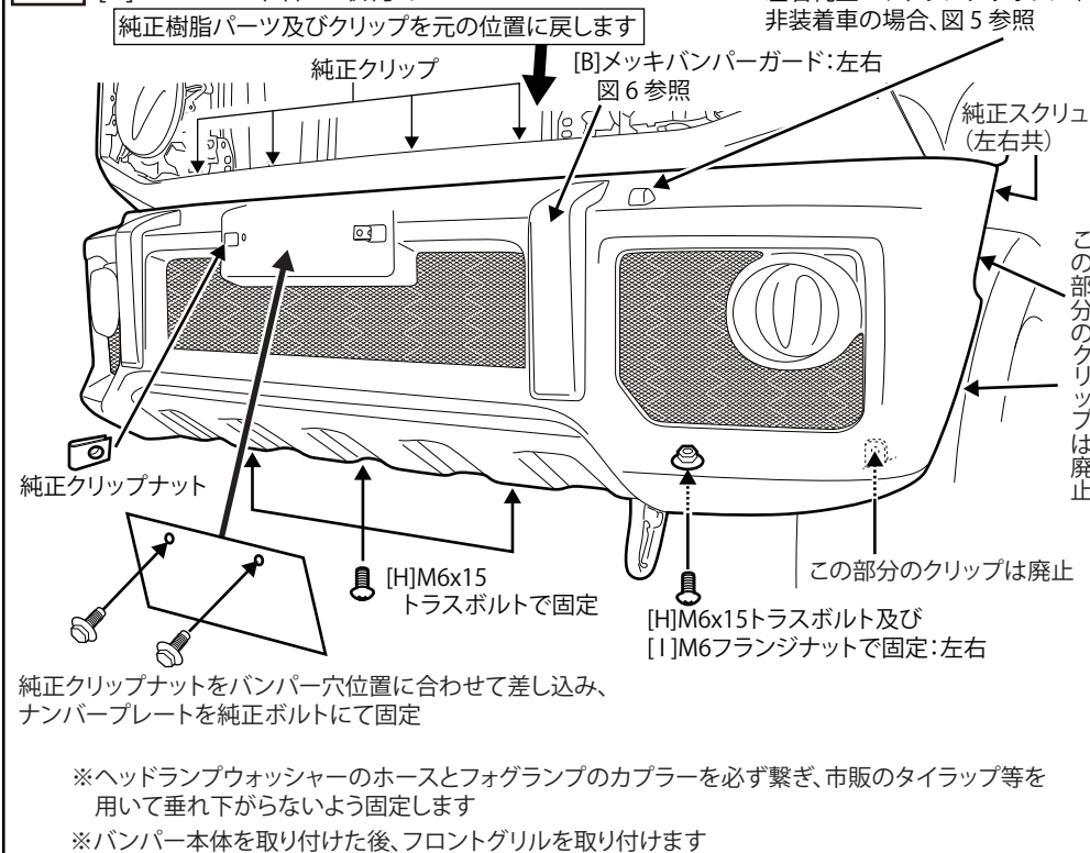
図4 [A]バンパー本体の取付け
